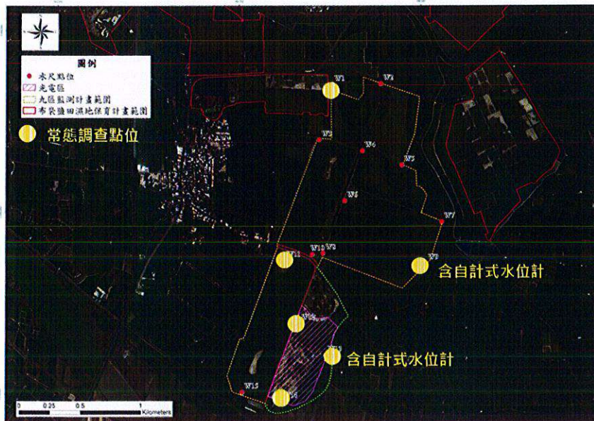
圖四、布袋鹽田第九區範圍施工後之水文調查之樣點示意圖
