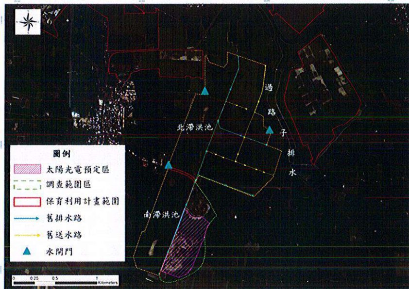
圖五、布袋鹽田第九區範圍內水路現況
